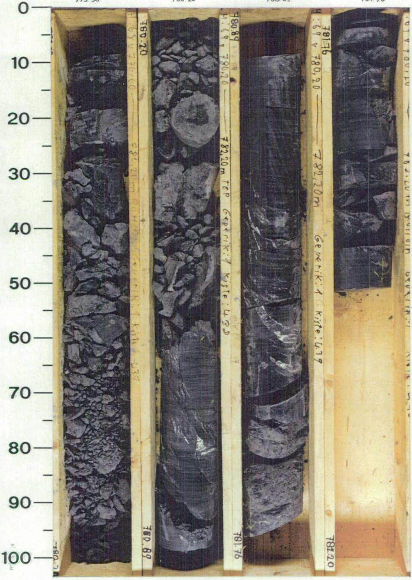
780.20 780.89 781.76 781.20 Kroon
