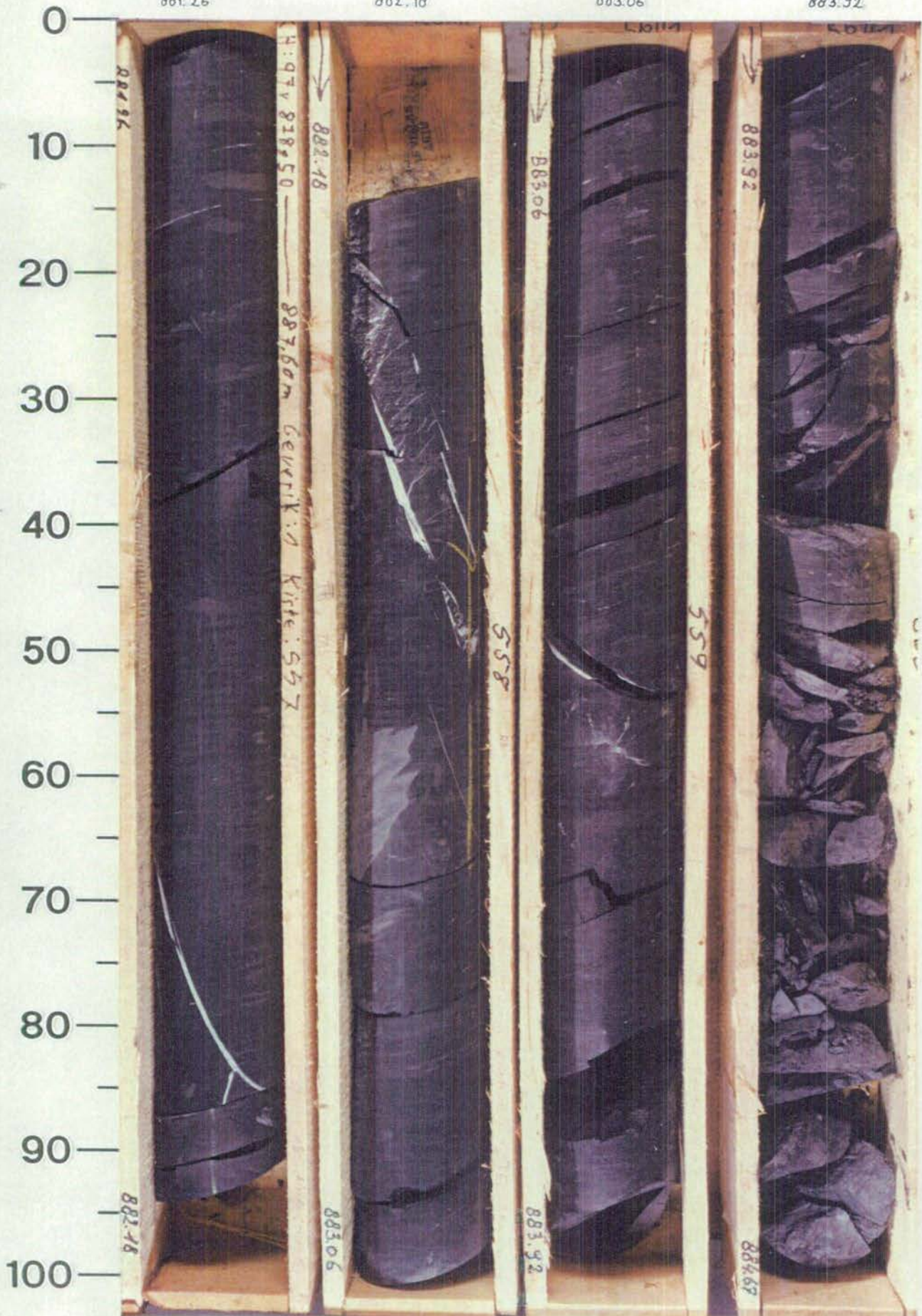
882.18 883.06 883.92 884.67 Kroon
